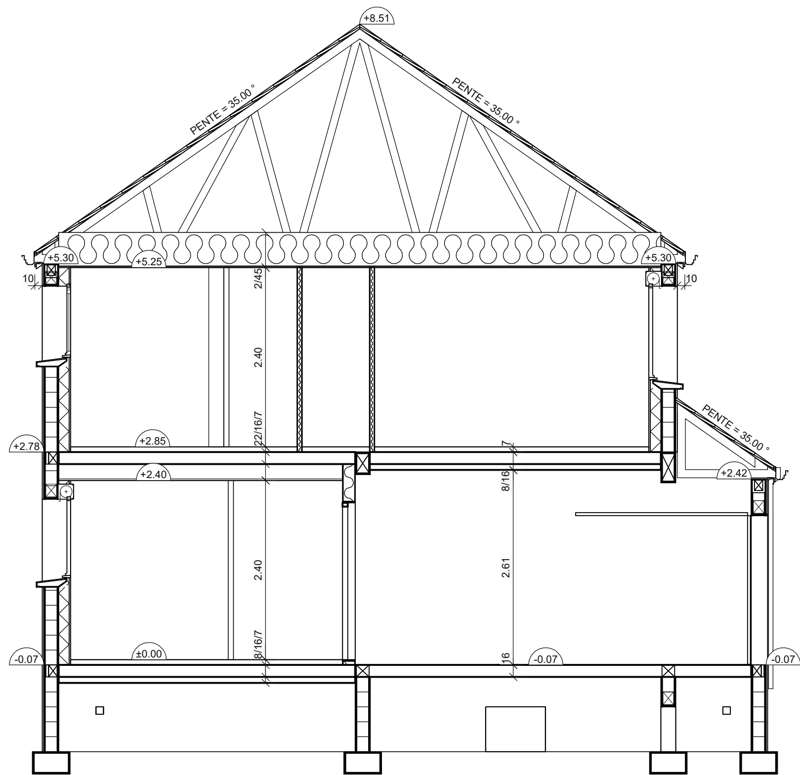
Coupe BB
