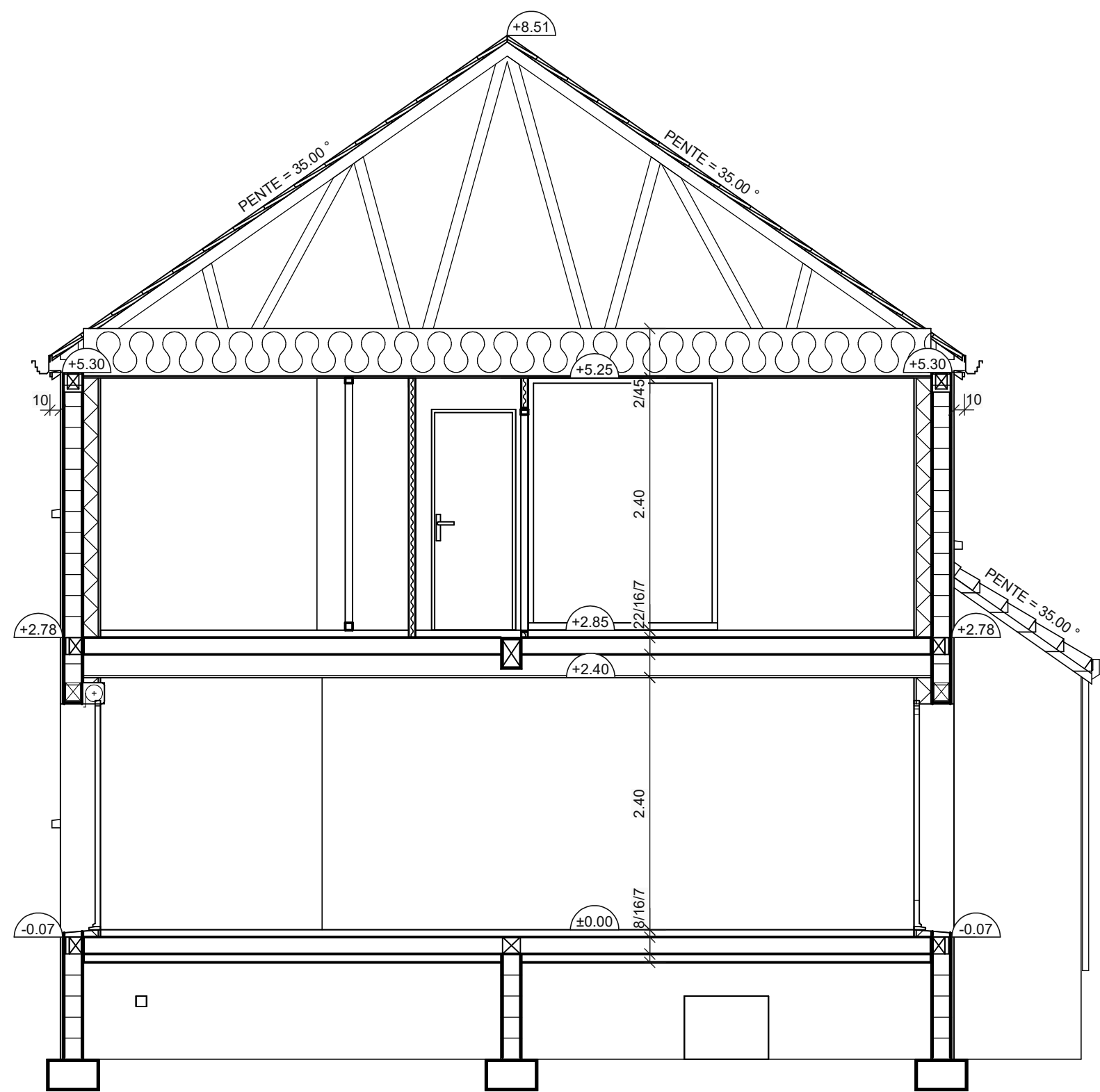
Coupe AA
