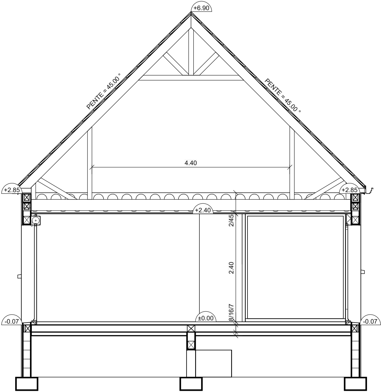
Coupe AA
